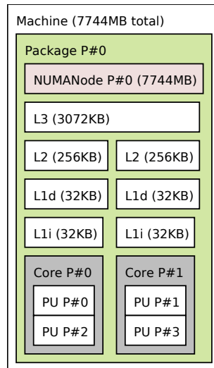
Σχήμα 3.1: Η τοπολογία ενός Intel® Core™ i3-7100U.
